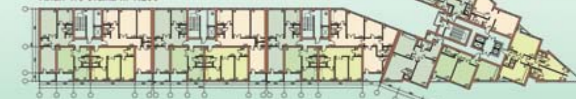
План типового этажа М 1:200
