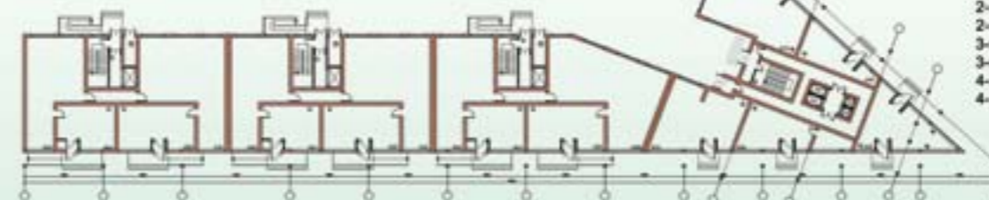
План 1го этажа М 1:200
