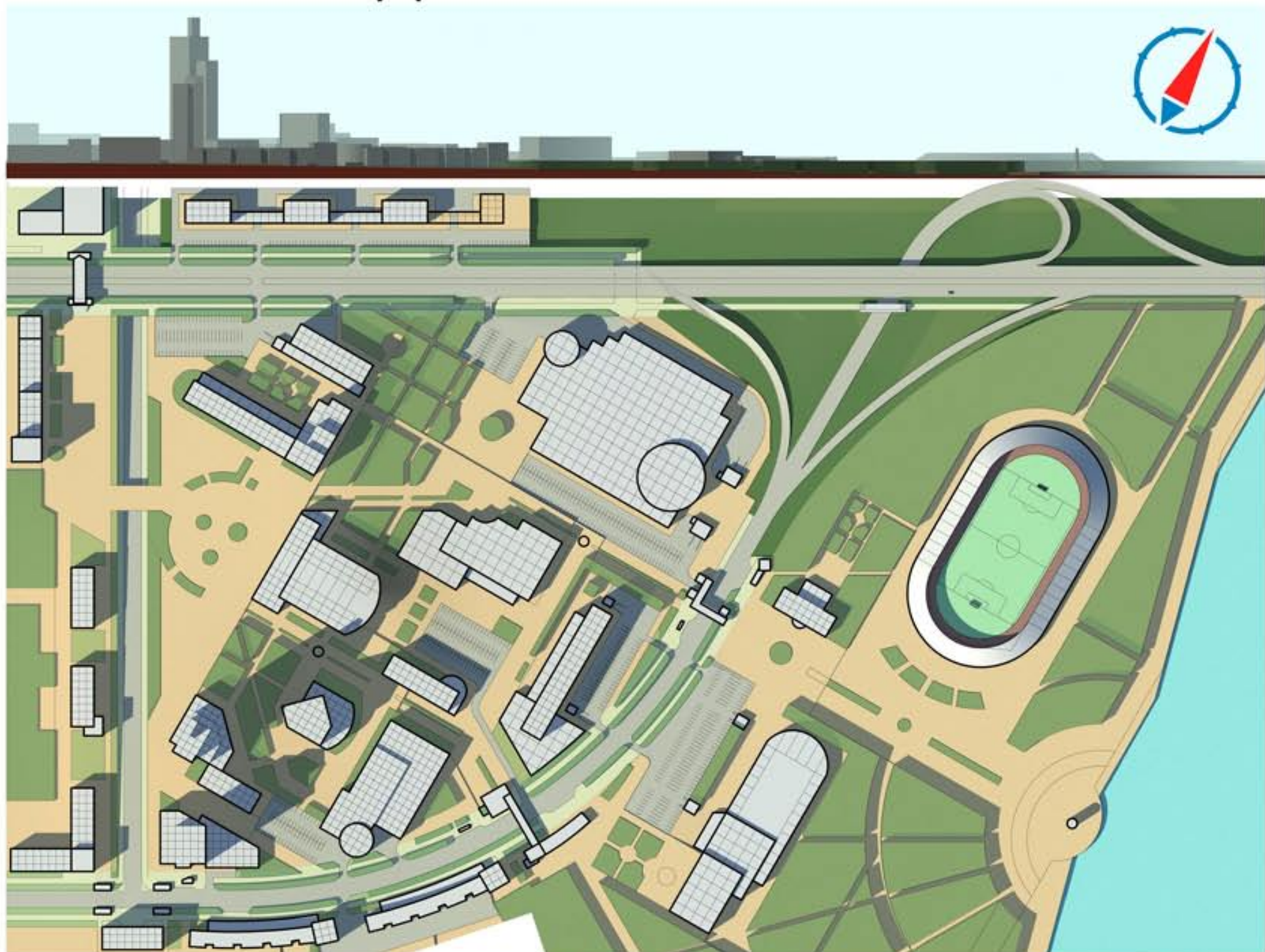
Генеральный план
