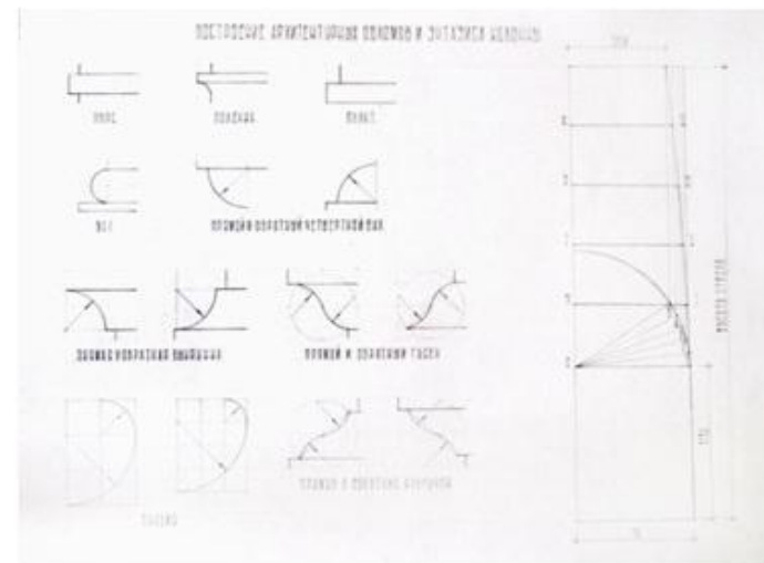
Построение коринфской капители и план базы (бумага, карандаш, 259x420)
