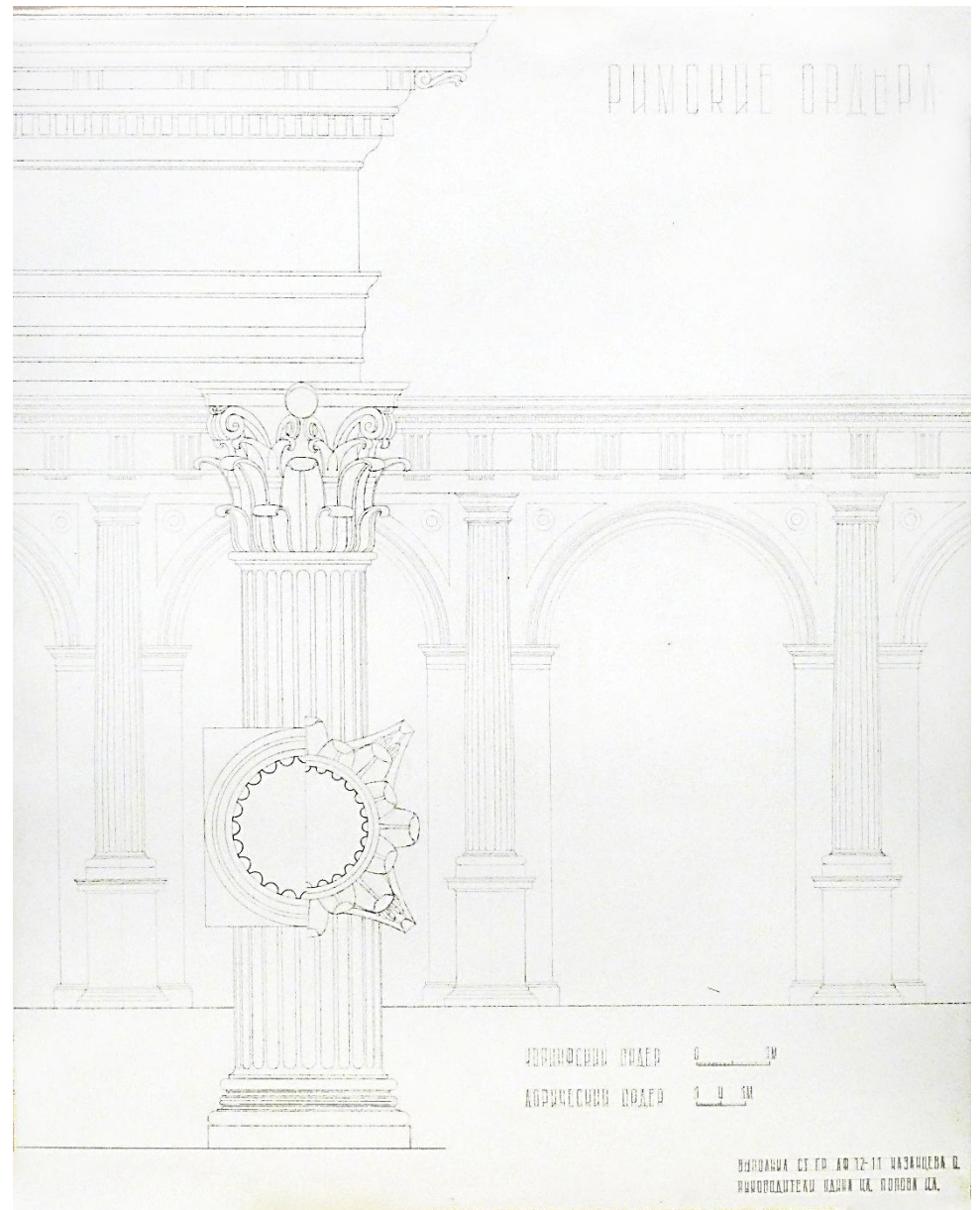
Павильон нерастанкино (бумага, тушь, перо, 75x55) Римские ордера (бумага, карандаш)
