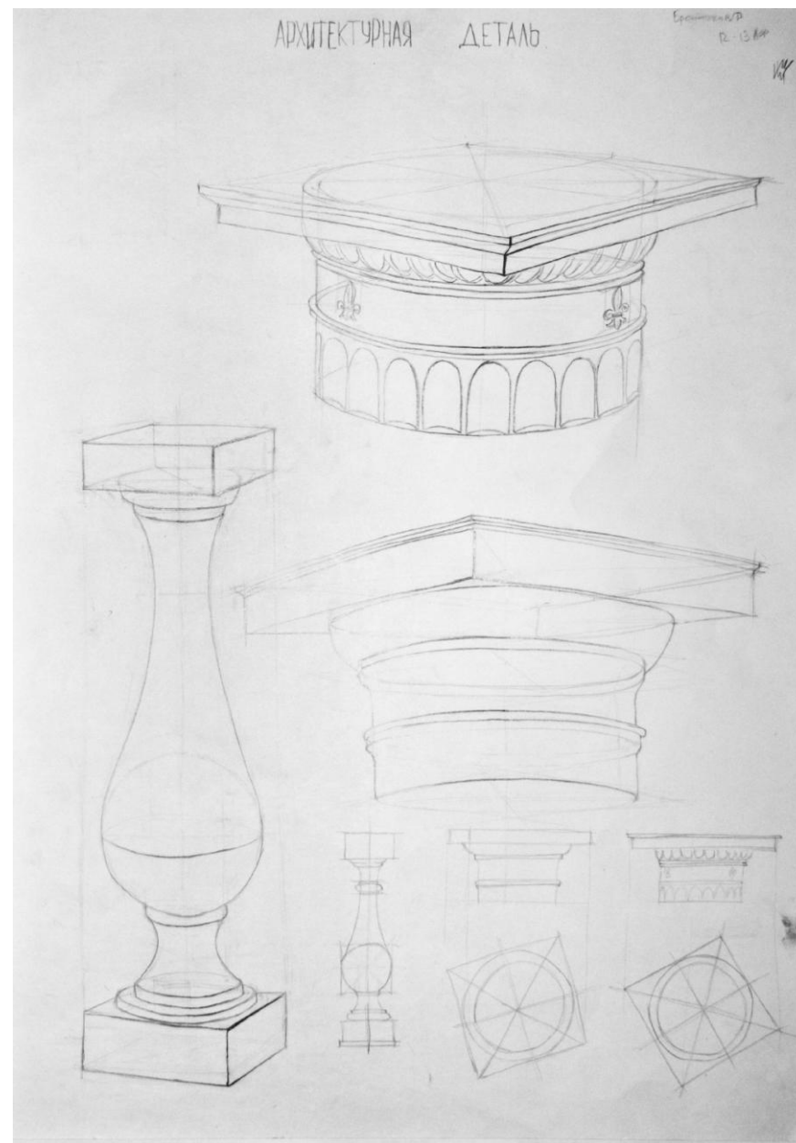
Архитектурная деталь (42 x 59,4, бумага, карандаш)
