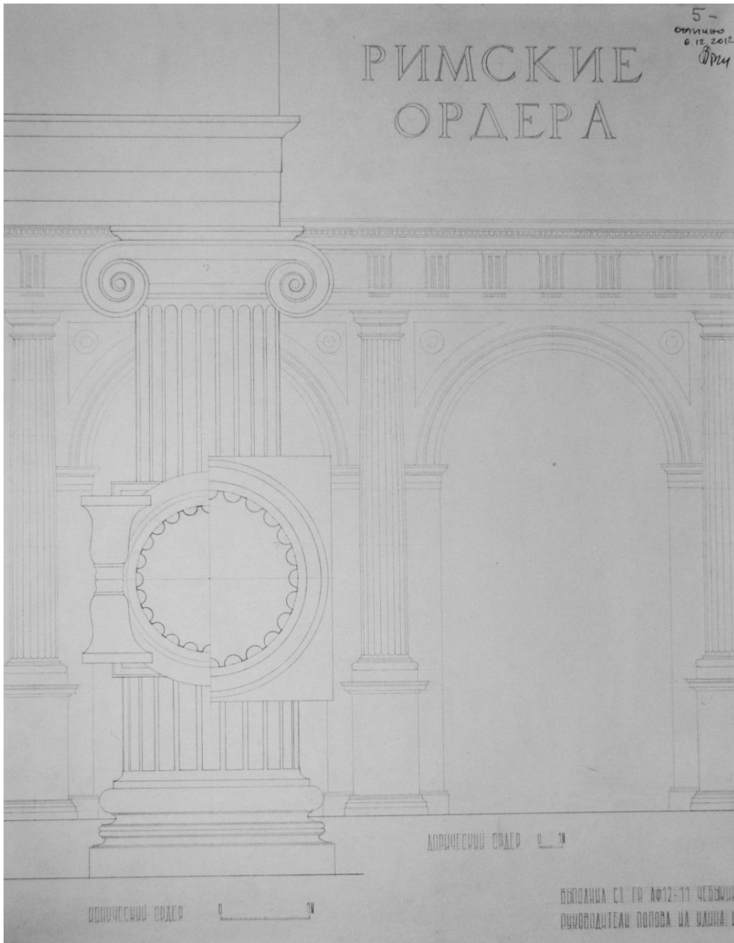
Римские ордера. Ионический и Коринфский ордер .( 55 x 75, бумага, карандаш)
