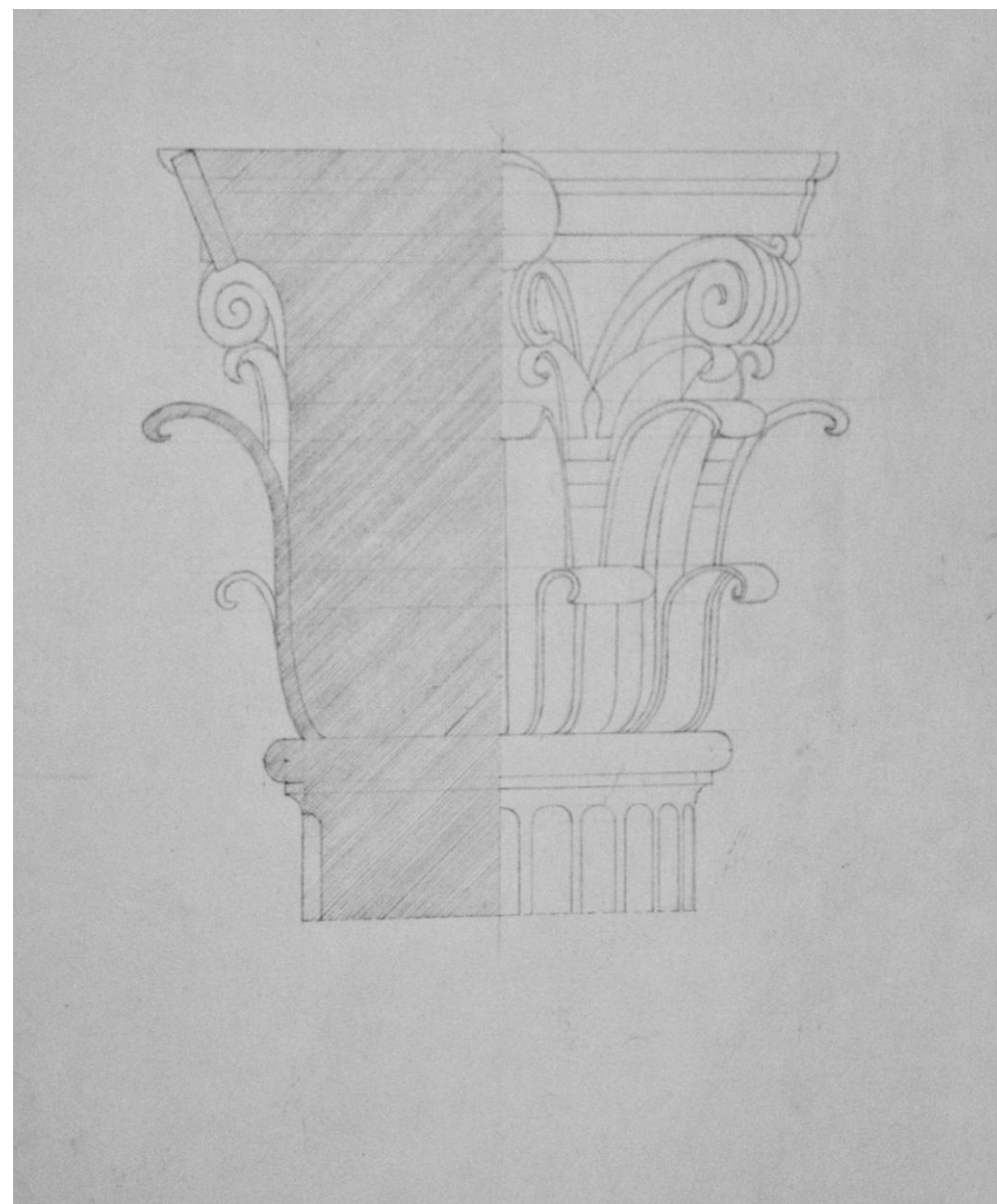
Построение капители коринфского ордера (29,7 x 42, бумага, карандаш) Построение архитектурных обломов (29,7 x 42, бумага, карандаш)
