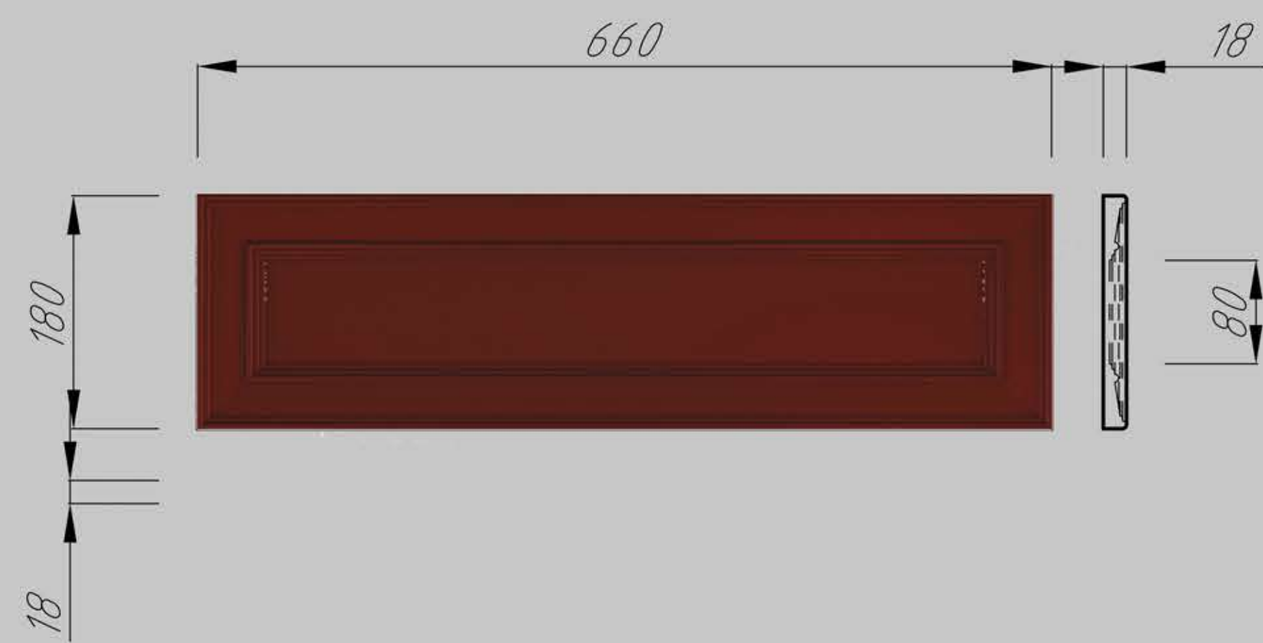
Дверца витрины М1:4
