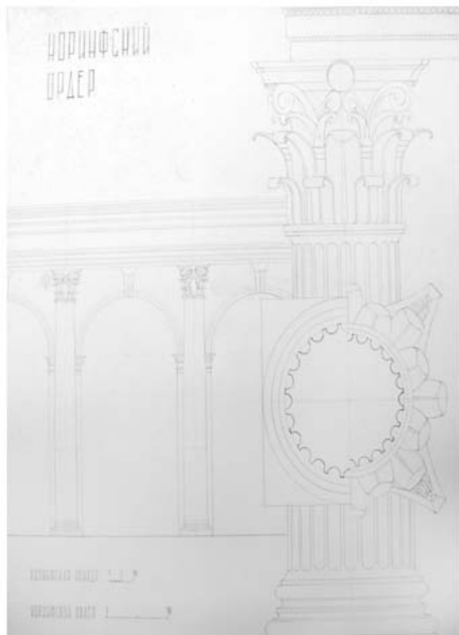
Проект. Коринфский ордер.
