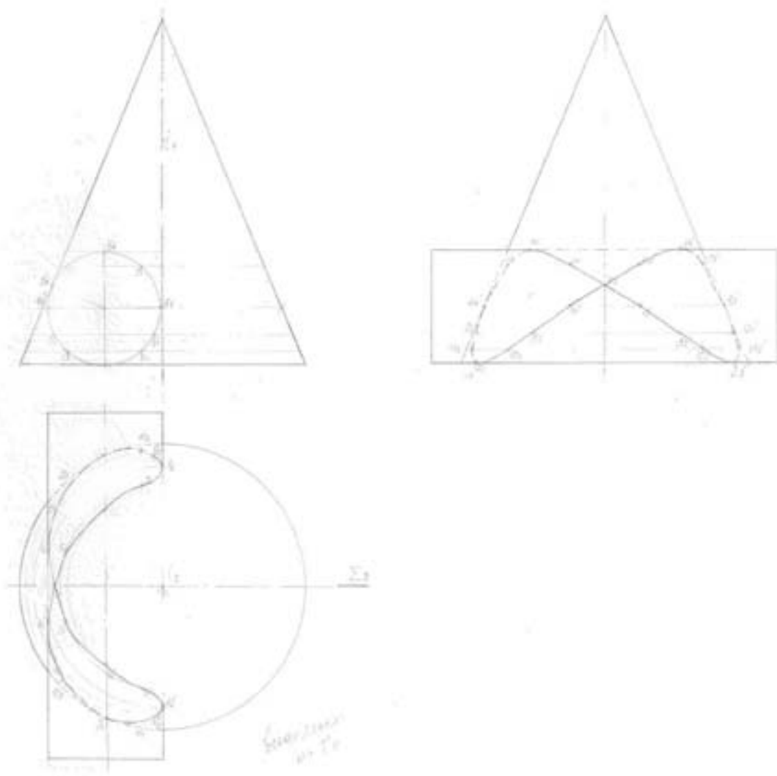
Пересечение поверхностей.
