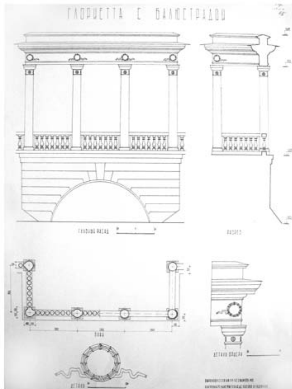
Проект. Глорietta с балюстрадой..
