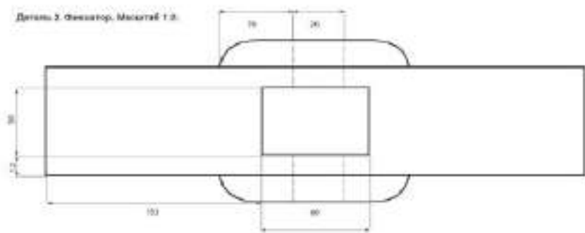
Деталь 2. Фюзеляж. Масштаб 1:3.
