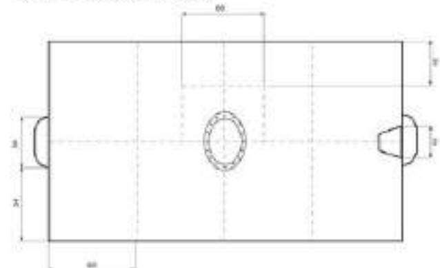
Деталь 1. Фюзеляж корабля. Масштаб 1:3.
