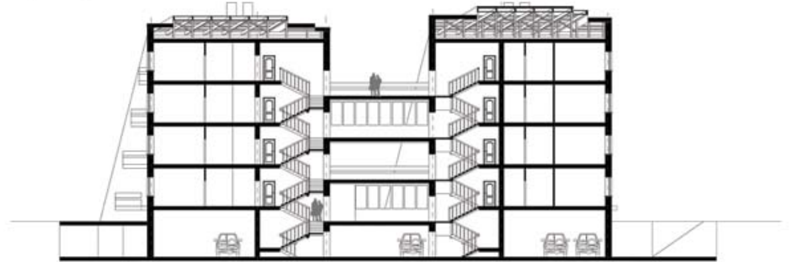
Жилой дом средней этажности, типовой этаж, разрез, 3 курс 6 семестр Das Wohnhaus mit mittlerer Geschößzahl, das typisierte Stockwerk, Schnitt, das 3. Studienjahr, das 6. Semester
