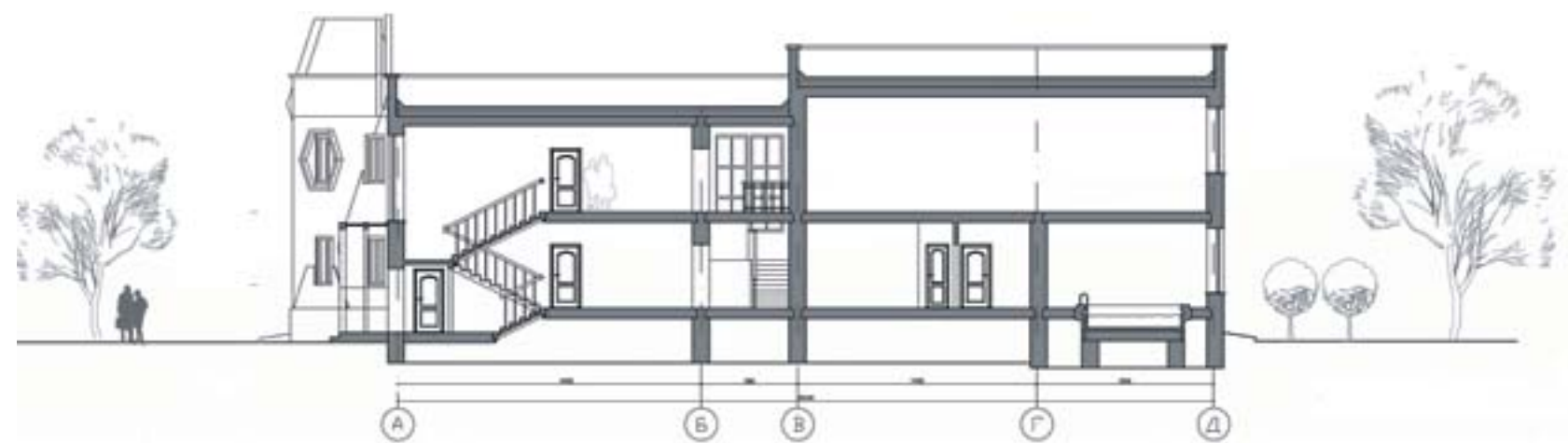
Детский сад на 4 группы, разрез, 3 курс 6 семестр Der Kindergarten auf 4 Gruppen, der Schnitt, das 3. Studienjahr, das 6. Semester > План 1 и 2 этажа, 3 курс 6 семестр Der Plan des 1. und 2. Stockwerkes, das 3. Studienjahr, das 6. Semester
