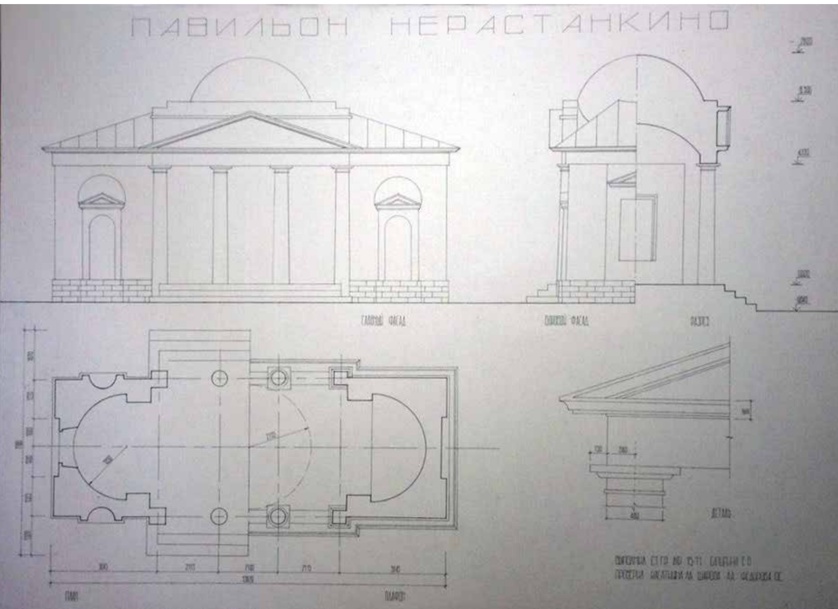
Павильон Нерастанкино в Царицыно Бумага, рапидограф. 2015г
