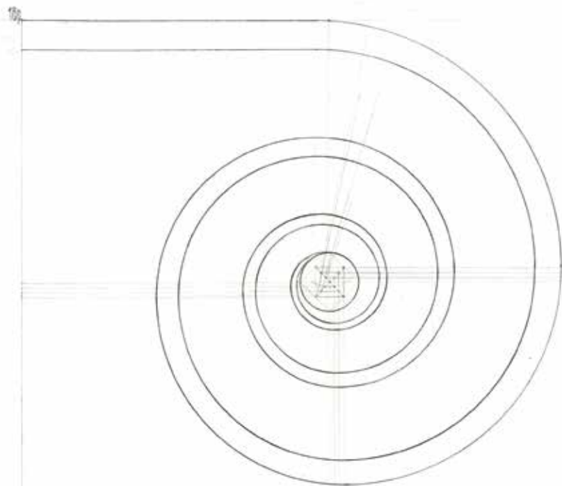
ПОСТРОЕНИЕ ВОЛЮТЫ 1 курс, 1 семестр бумага, карандаш 2016
